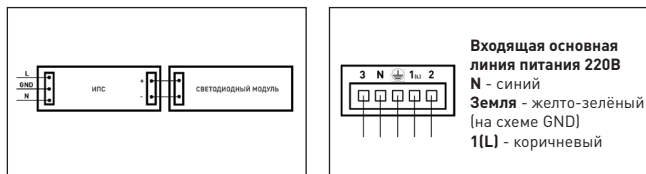
Схема электрическая
