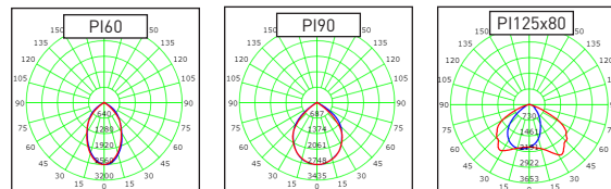
Диаграммы кривых силы света
