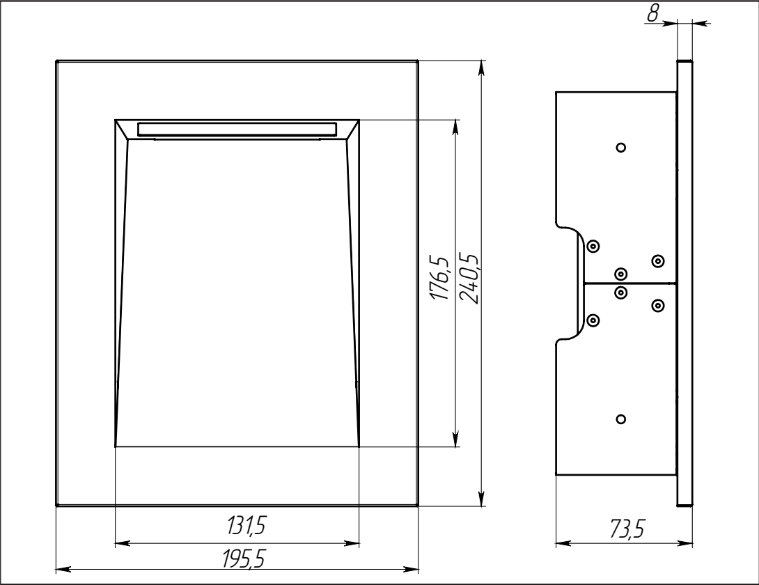
Габаритные размеры светильника
