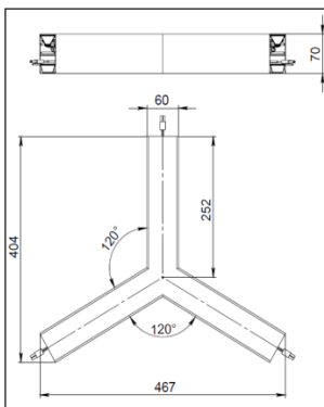
FORM-Y 120- образное 120°
